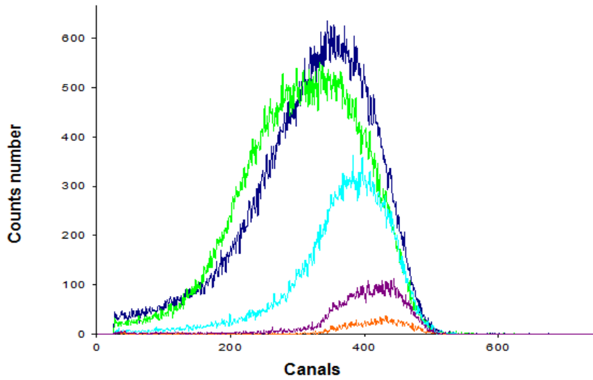
Fig. 4. ERDA spectra of V1, V2, V3, V4 and V5 glasses
